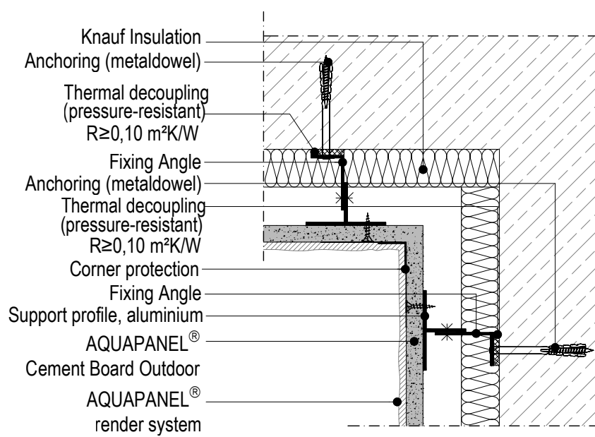
KNAUF W684T-D1.en Inner corner
