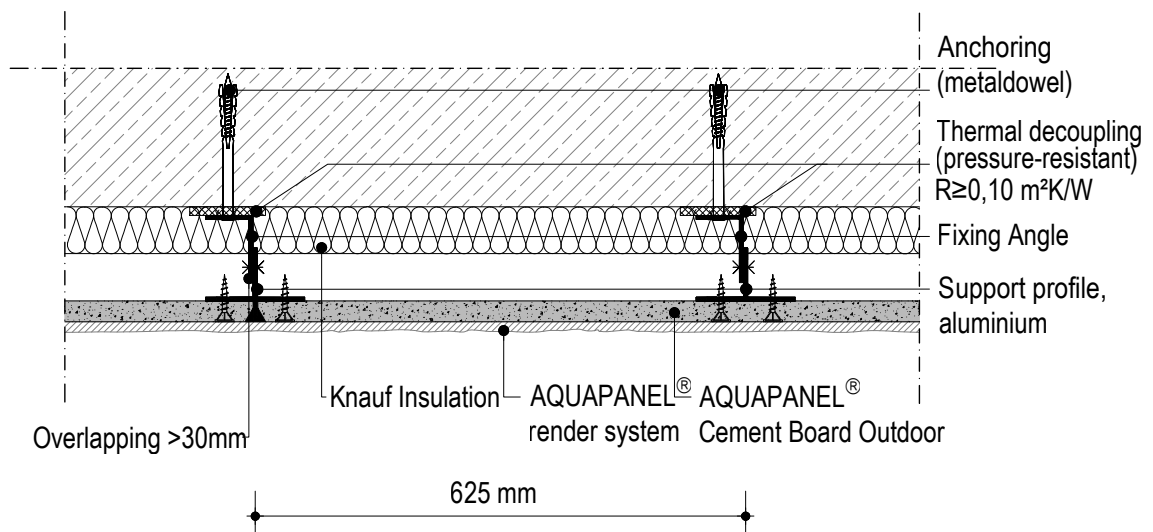
KNAUF W684T-H1.en Horizontal section
