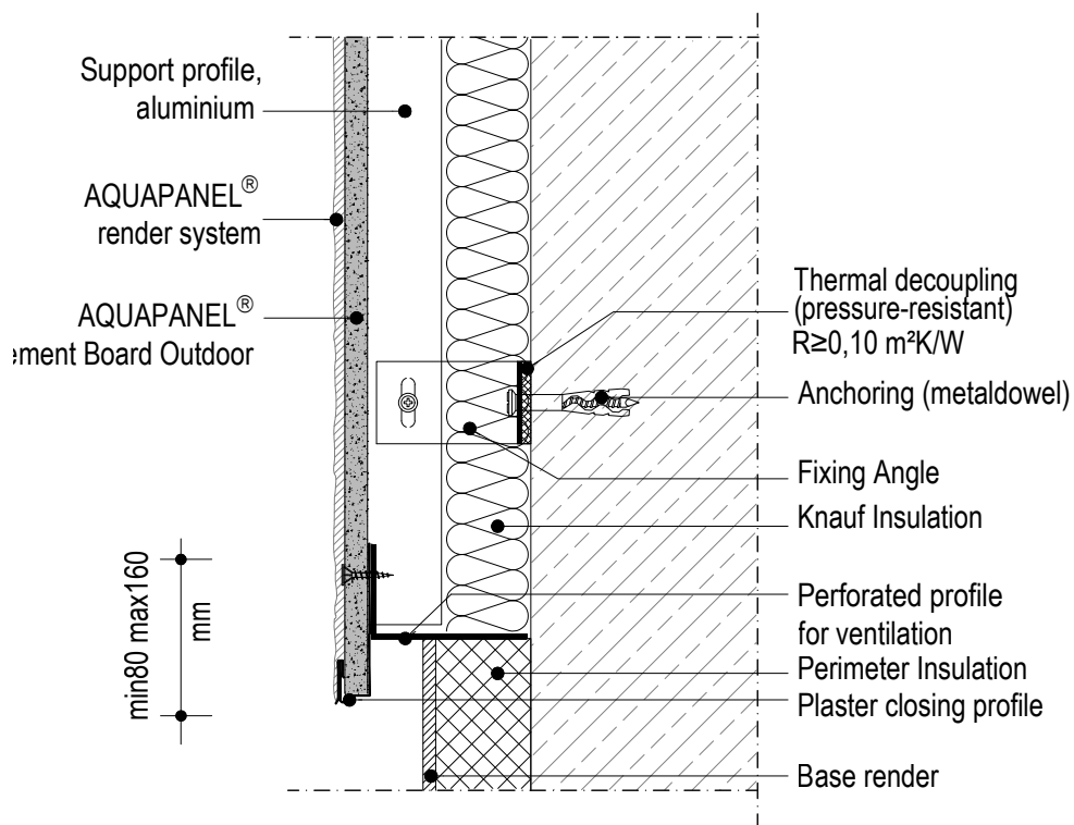
KNAUF W684T-SO-V1.enFoot point, Option 2
