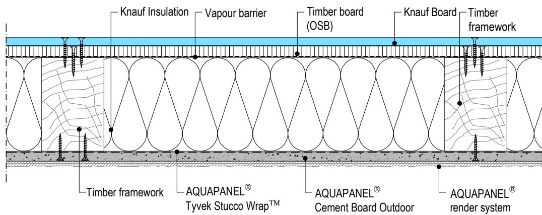
knauf W571-H1.en Horizontal Section
