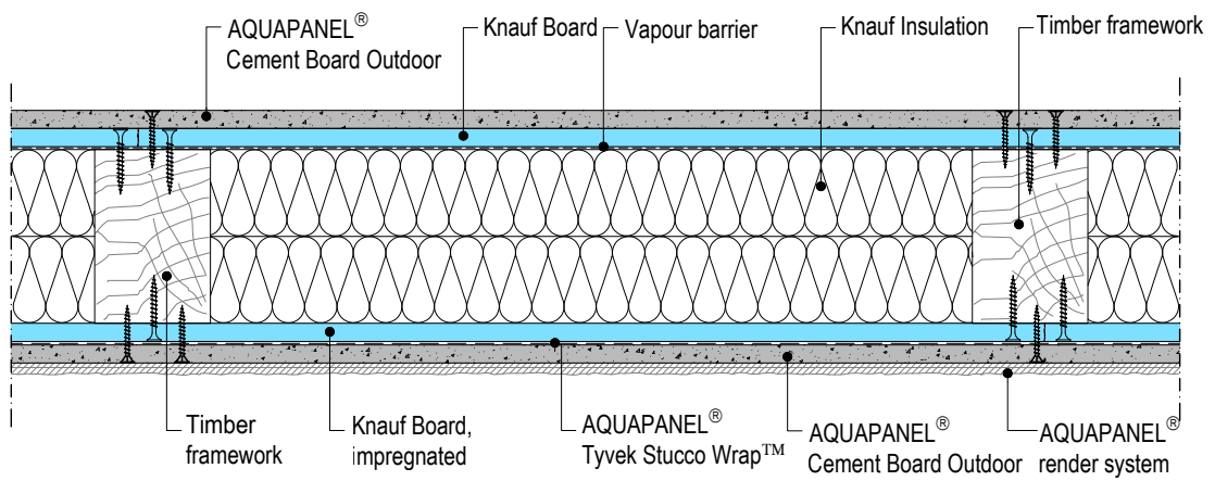
knauf W572-H1.en Horizontal Section
