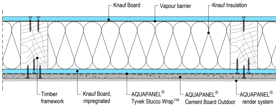
KNAUF W572-H2.en Horizontal Section
