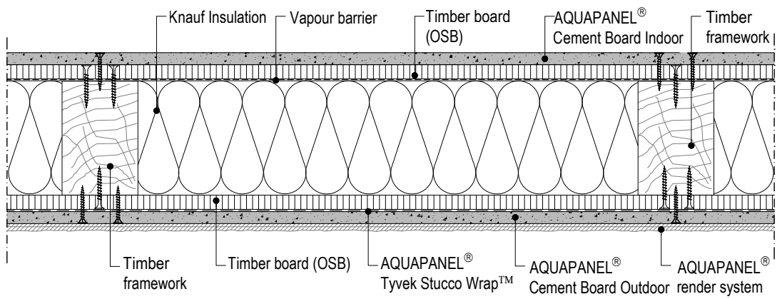
KNAUF W573-H1.en Horizontal Section
